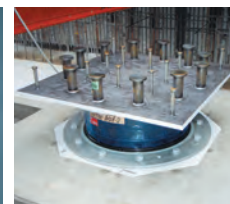
免震装置
