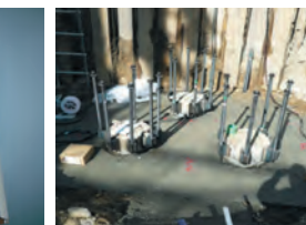
クラウンパイルアンカー
