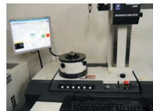
真円度測定器
